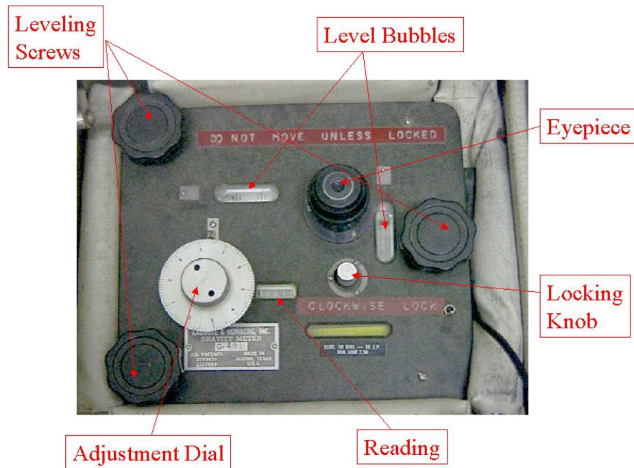
Worden Gravity Meter
